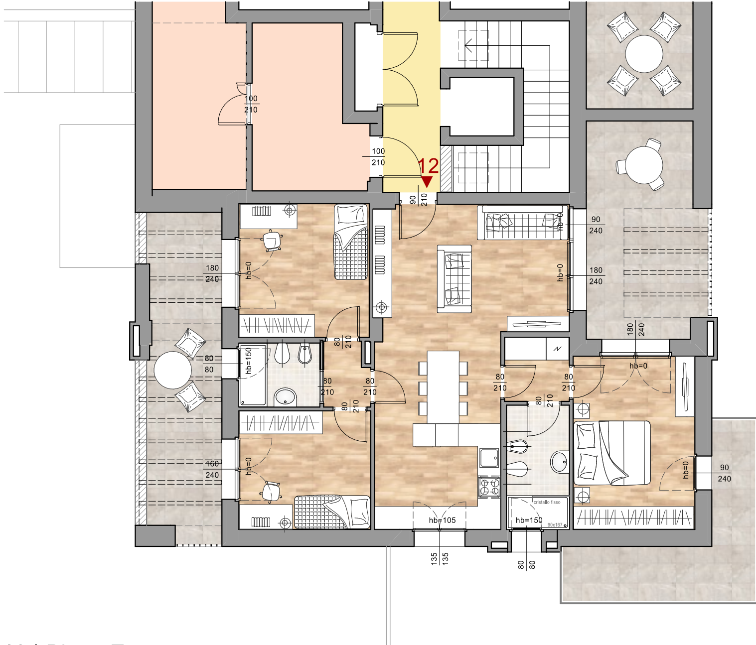
ALLOGGIO 12 | Piano Terzo Scala 1:100
